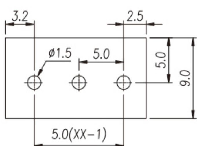
P.C.B. LAYOUT
