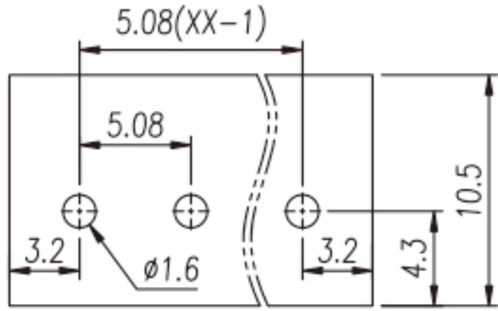
P.C.B. LAYOUT
